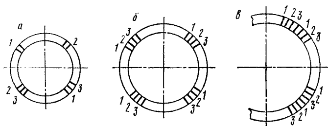
Рис. 3. Схема вырезки образцов для механических испытаний
