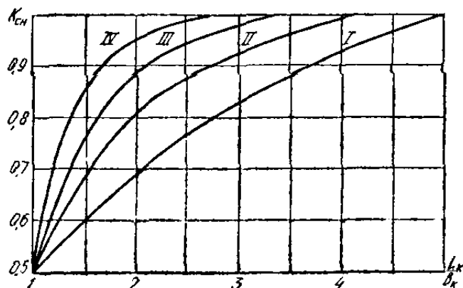
Рис. 6. Графики для определения коэффициента k_{сн} L_k - длина камеры; B_k - ширина камеры, I, II, III, IV - категории
