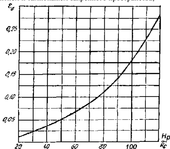
Рис. 3. График для определения \varepsilon_0
