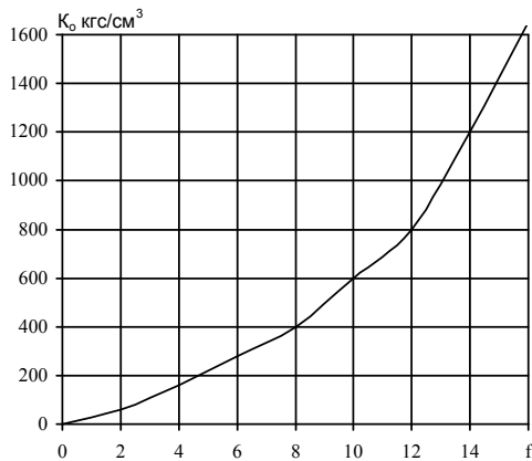
Черт. 2. График зависимости коэффициента K_0 от коэффициента крепости грунта f для трещиноватых грунтов
