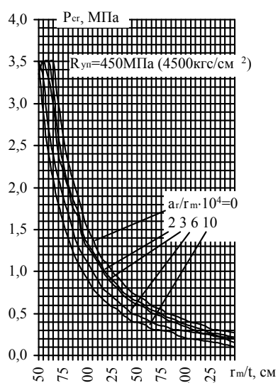
Черт. 2. График зависимости критического наружного давления \rho_{cr} от относительной толщины стенки r_m/t [ R_{yn} – нормативное сопротивление по пределу текучести стали, МПа ( \text{кгс}/\text{см}^2 ); a_r – расчетный радиальный зазор между стенкой оболочки и бетоном, см; r_m – средний радиус оболочки, см; t – толщина стенки оболочки, см]
