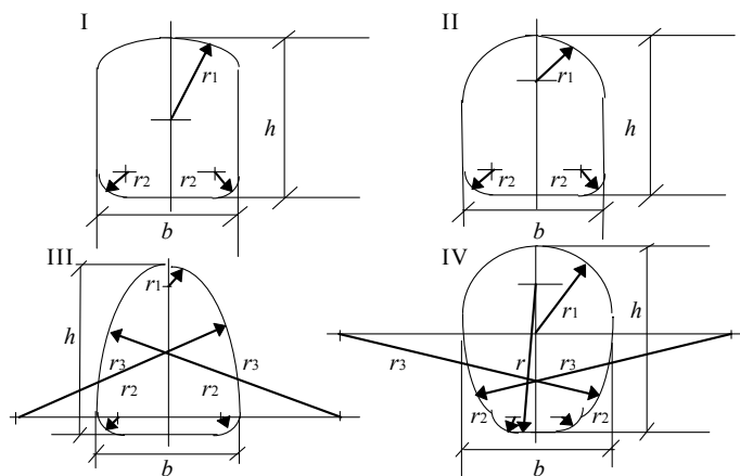
Черт. 1. Формы поперечных сечений безнапорных туннелей в свету
