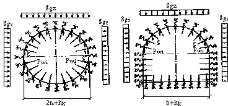
Черт. 1. Расчетные схемы обделок туннелей
