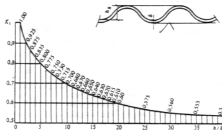
Черт.7. График для определения коэффициента K_l
