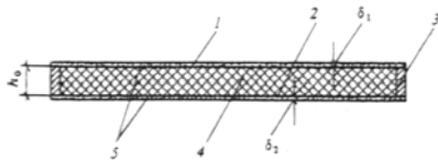
Черт.5. Поперечное сечение бескаркасной панели с обрамлением 1, 2 - асбестоцементные обшивки; 3 - элементы обрамления панели; 4 - заполнитель (пенопласт); 5 - клеевой шов.
